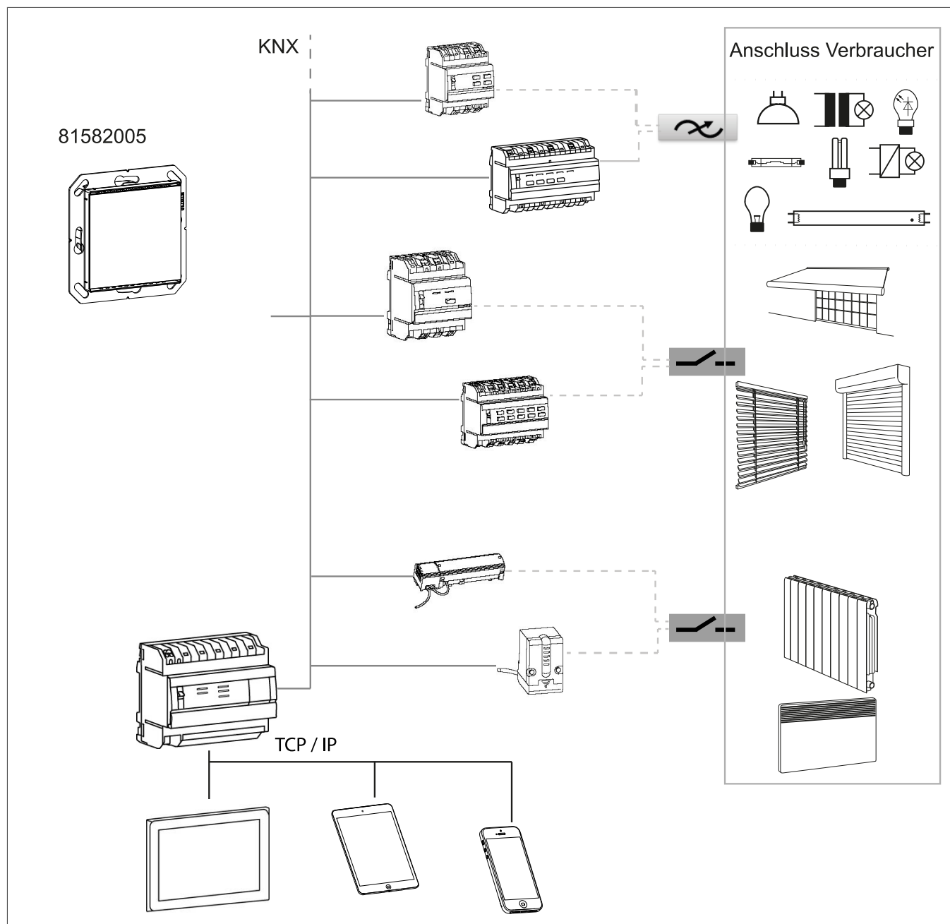
Abbildung 1: Geräteübersicht
