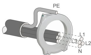
Fig. 9: Distribuzione via cavo
