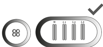
Fig. 7: Distribuzione corretta dei cavi
