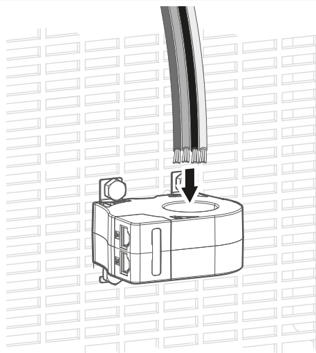
Fig. 6: HR72x - Passaggio dei cavi
