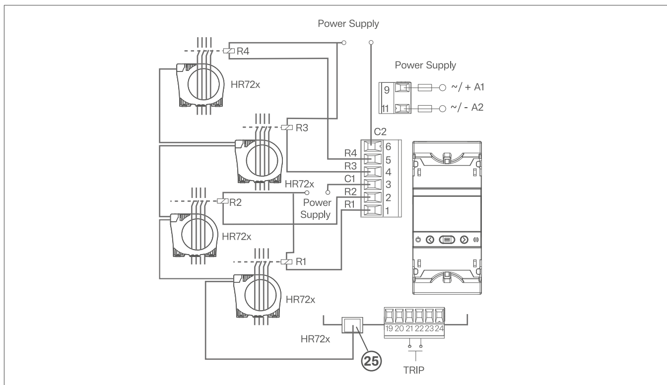
Fig. 14: HR554 - Collegamento elettrico
