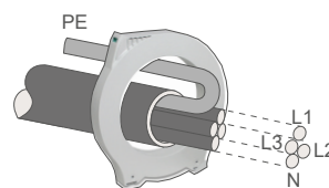
Fig. 10: Distribuzione dei cavi (canalina)
