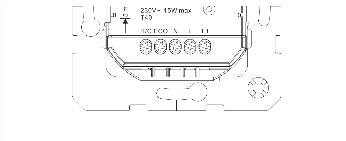
Bild 3: Detailansicht Anschlussklemmen
