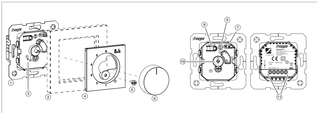
Bild 2: Geräteaufbau
