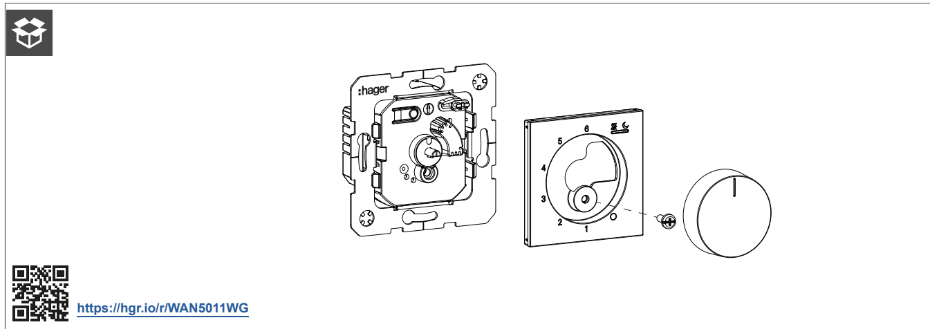
Bild 1: Lieferumfang WAN5011xx
