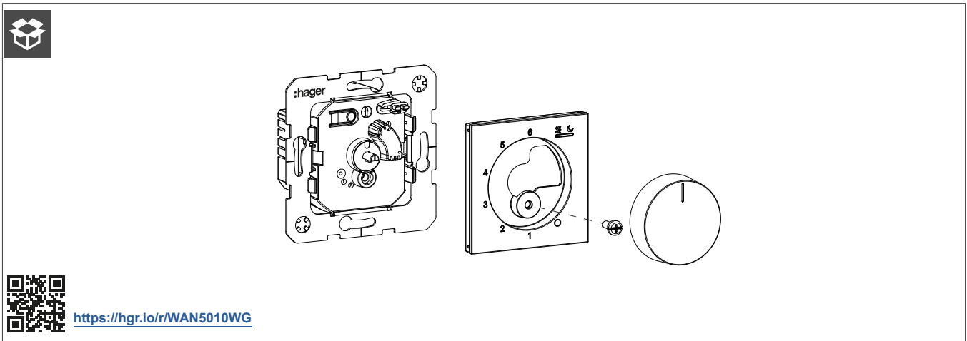
Bild 1: Lieferumfang WAN5010xx
