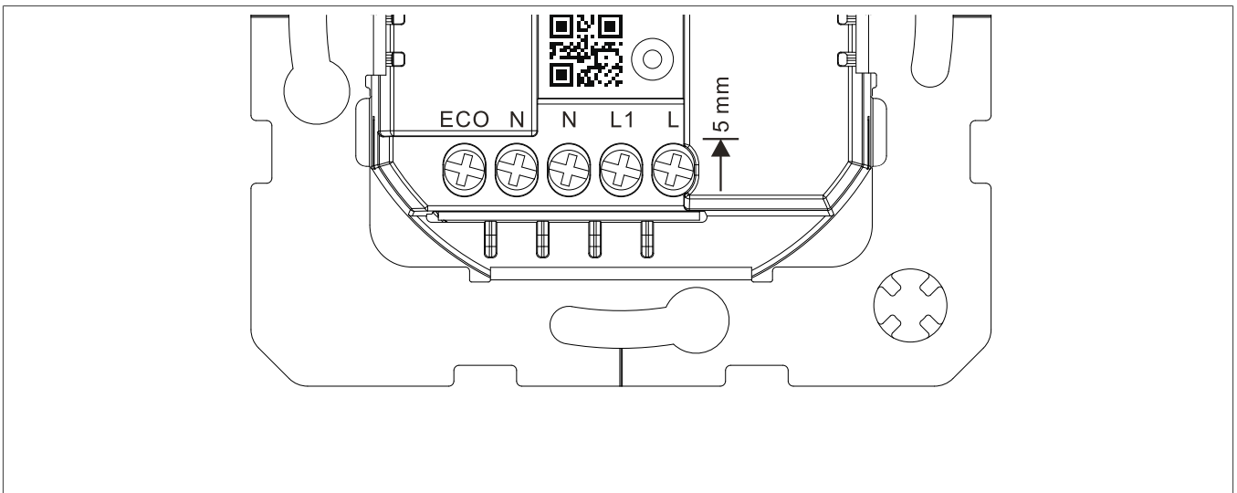
Bild 3: Detailsicht Anschlussklemmen
