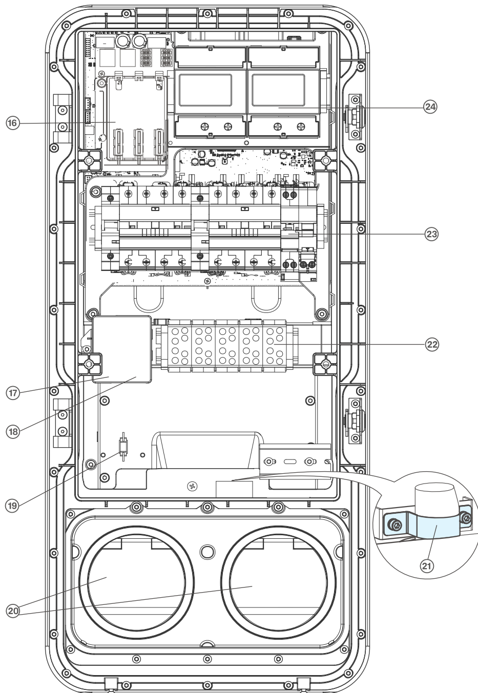
Bild 8: Gerätesockel
