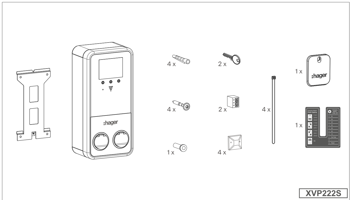
Bild 1: Lieferumfang für Ladestation witty park 2 2x 22kW T2S Wandmontage
