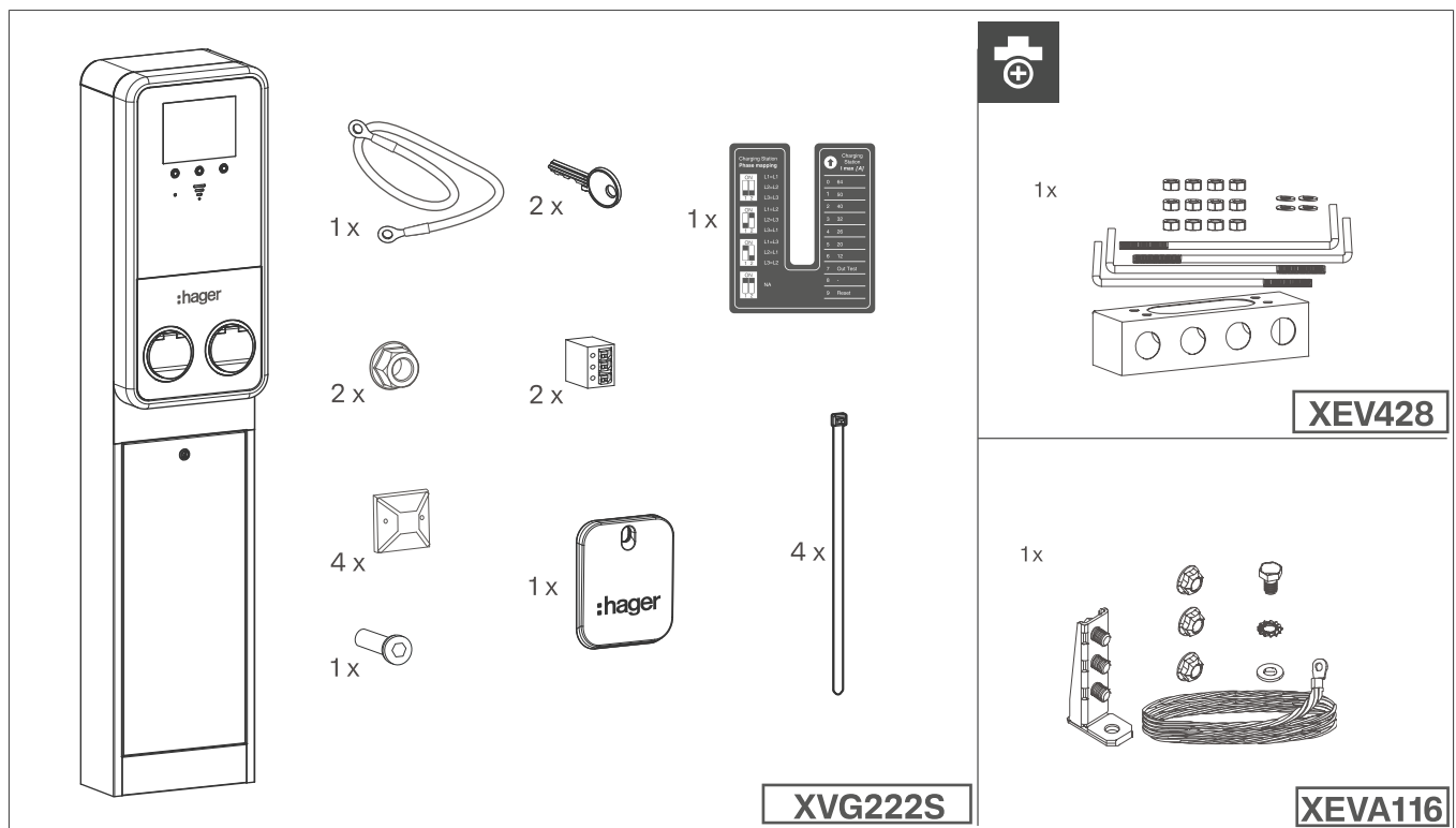
Bild 2: Lieferumfang für Ladestation witty park 2 x 22kW T2S Freistehend
