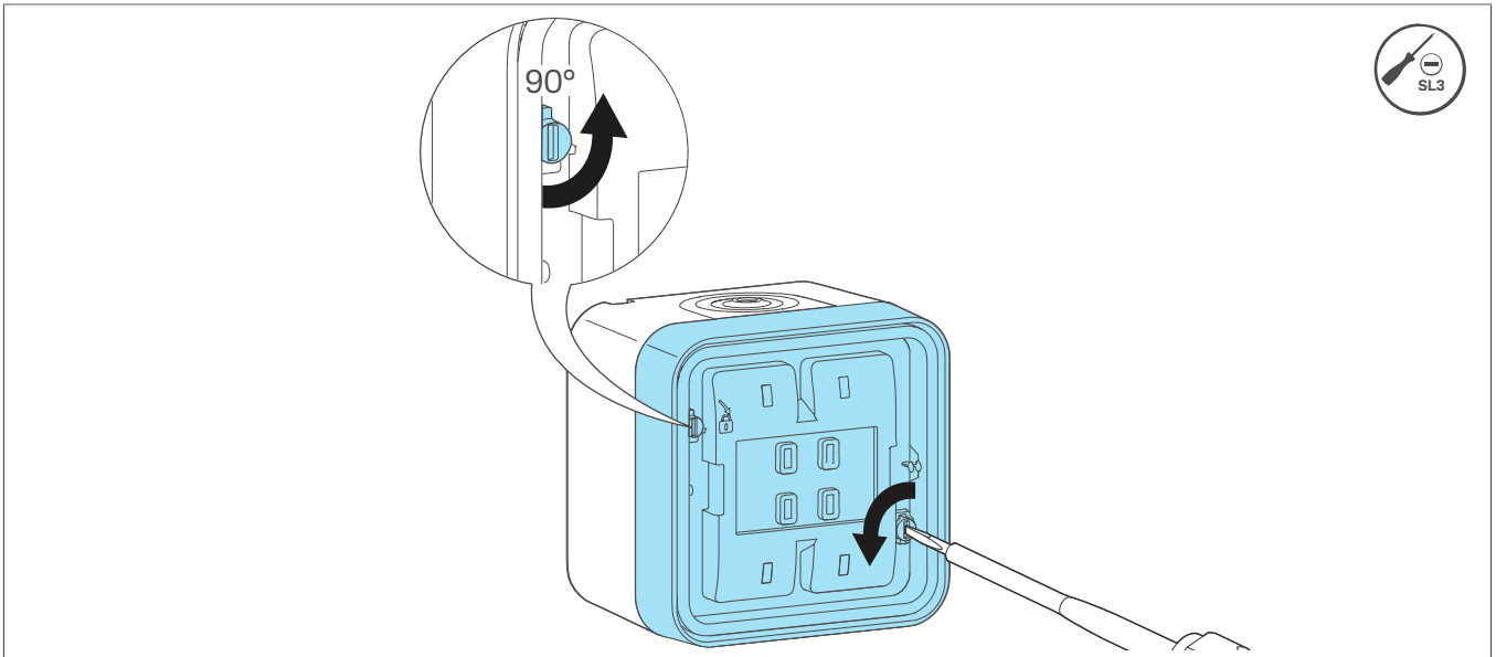
Afbeelding 3: Ontgrendel de connectors met bajonetting
