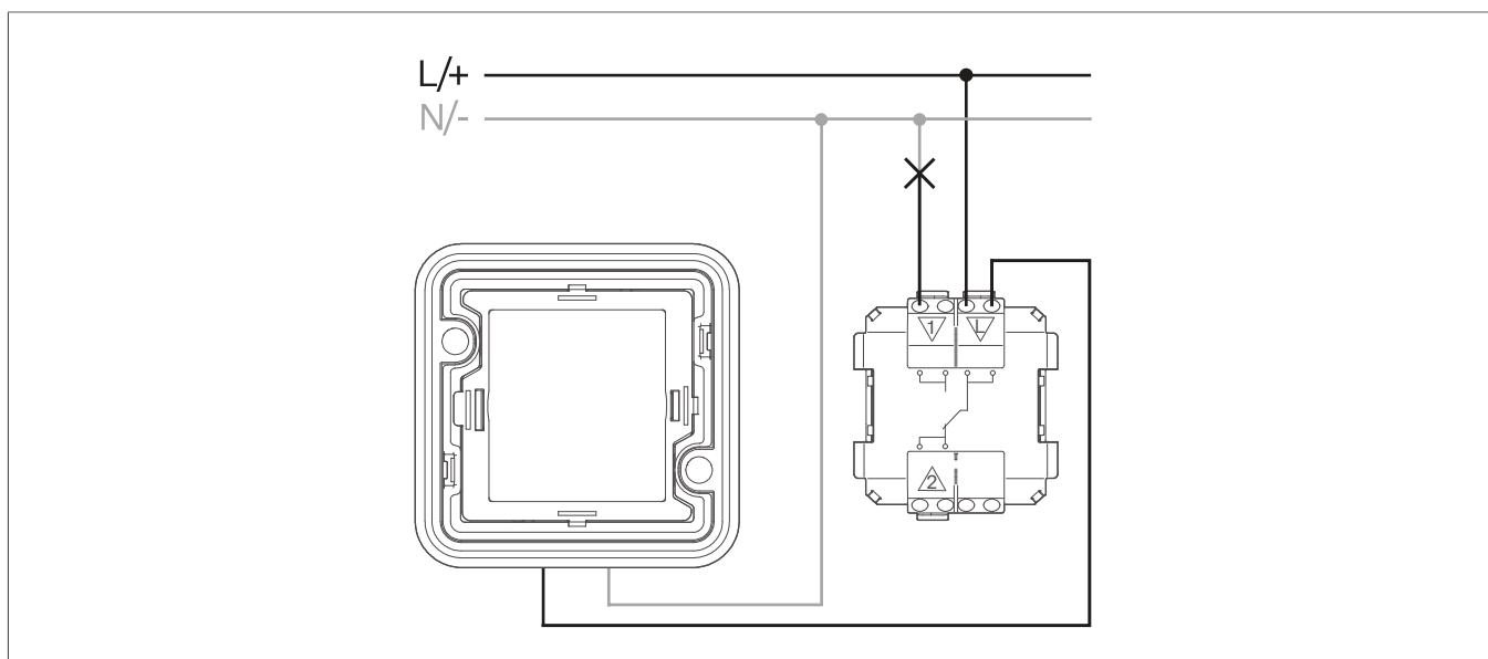
Afbeelding 6: Aansluitschema voor permanente verlichting
