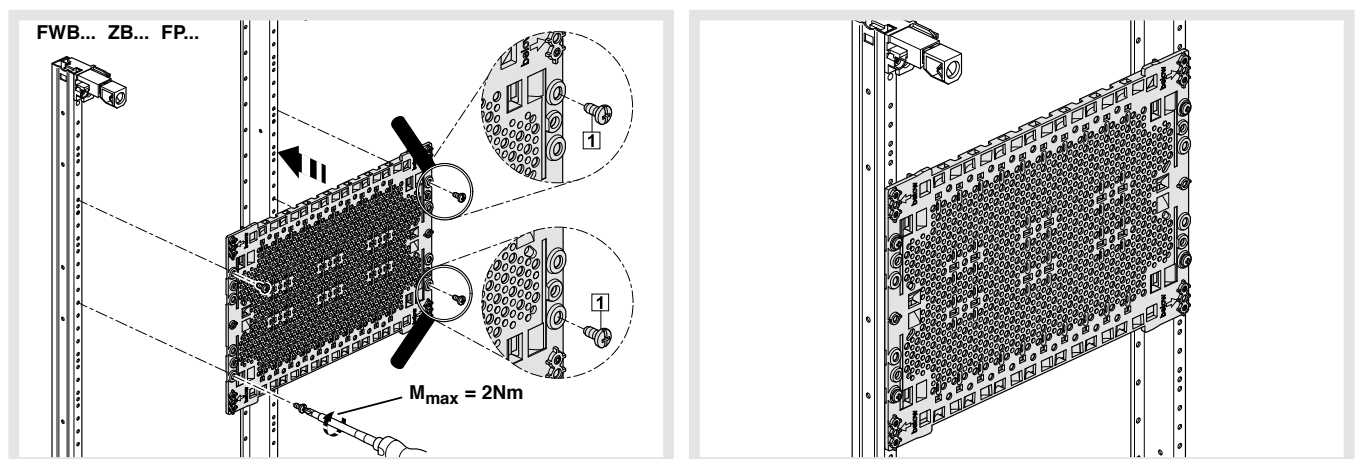
Montage der Kunststoff-Montageplatte UM00M0 auf der Vorderseite der univers Z Tragschienen
