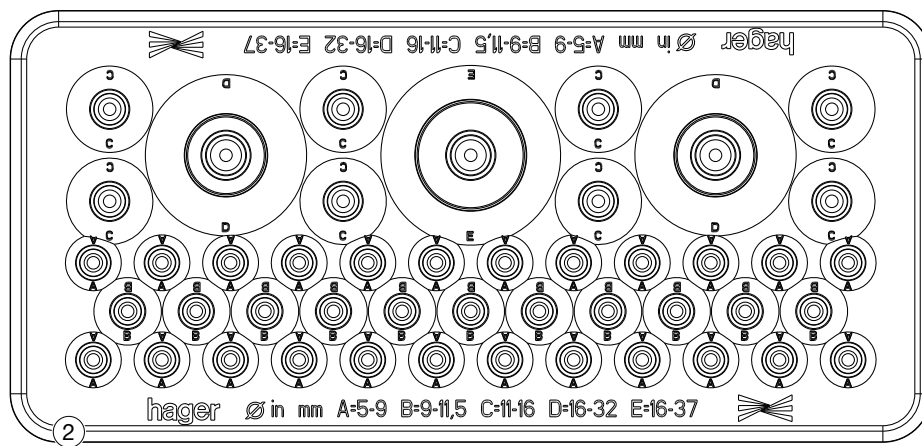
Lochbild der oberen/unteren Leitungseinführungsflansch FZ426
