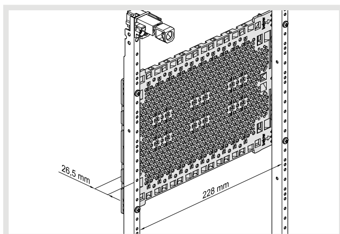
Montage der Kunststoff-Montageplatte UM00M0 auf der Rückseite der univers FW Tragschienen
