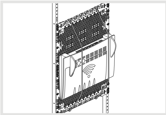
Befestigungssatz VZ340 mit Modem montiert an Montageplatte UM00M0
