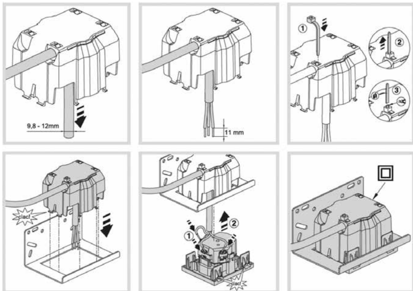
Montage des Deckels WH37961523Z für FLF-Steckdosen Gr. II zur Gewährleistung der Schutzklasse II
