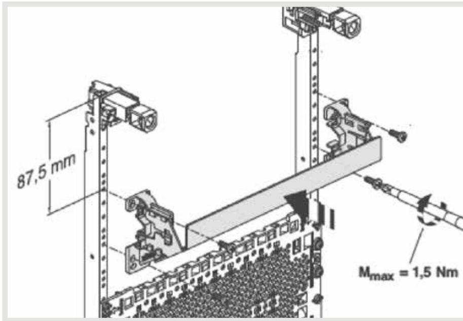
Montage der Abdeckung für Patchpanel-Träger Volta FZ12MM
