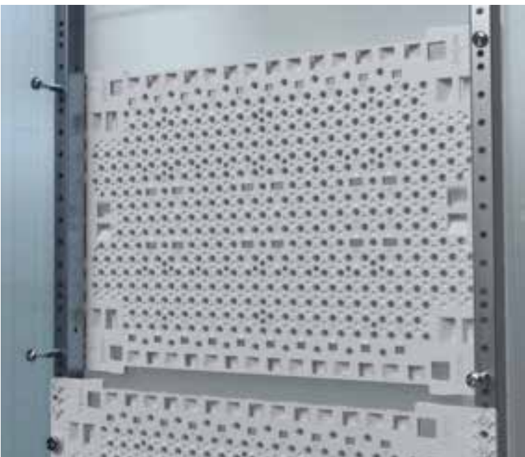
Montageplatte auf Rückseite der univers FW Tragschienen (oben im Bild) Montage auf Vorderseite der univers FW Tragschienen (unten im Bild)
