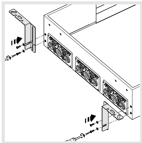
Montage von Befestigungslaschen-Set FZ900 für Unterputz- oder teilversenkten Einbau
