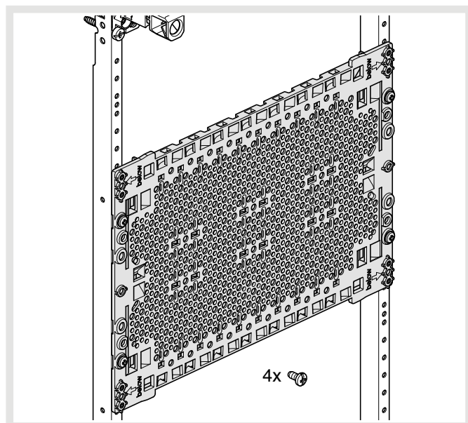
Montage der Kunststoff-Montageplatte in UMx1UK
