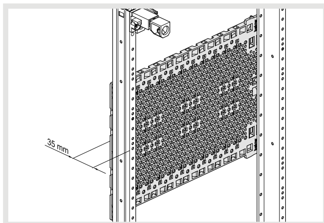
Montage der Kunststoff-Montageplatte UM00M0 auf der Rückseite der univers Z Tragschienen
