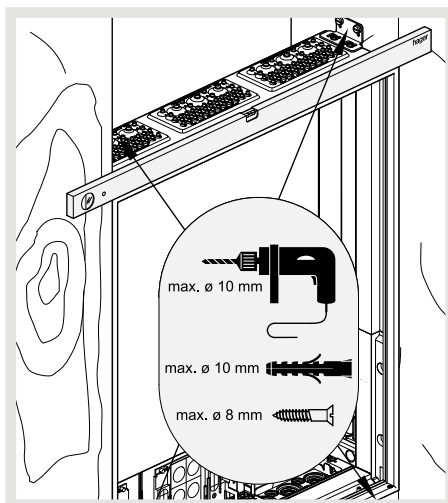
Montage von Befestigungslaschen-Set FZ900H für Unterputz- oder teilversenkten Einbau
