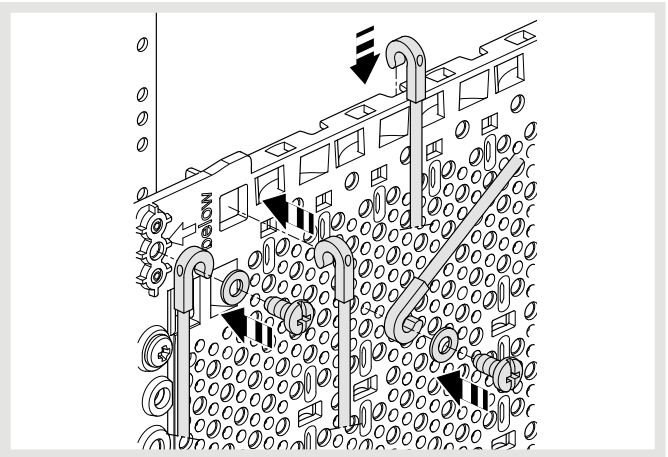
Montageoptionen für Befestigungssatz VZ340
