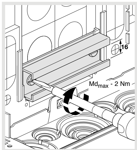
Befestigung von dickem Rohr am Schrank Kunststoff-Fußteil
