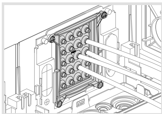
Schrank mit montierter Flansch FZ428 am Kunststoff-Fußteil (Ansicht von vorne)
