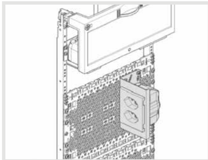
Montage des Steckdosenhalters UM00H0 auf Montageplatte
