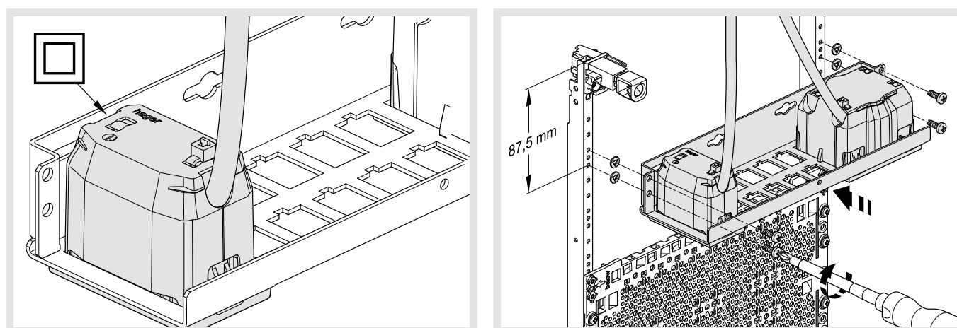
Montage des Deckels WH37961623Z für FLF-Steckdosen Gr. I zur Gewährleistung der Schutzklasse II
