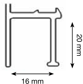
Integrierter Kabelkanal im mittleren Bereich unterhalb der Tragschiene
