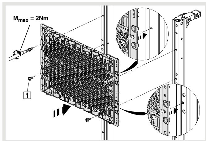
Montage der Kunststoff-Montageplatte UM00M0 auf der Rückseite der univers Z Tragschienen
