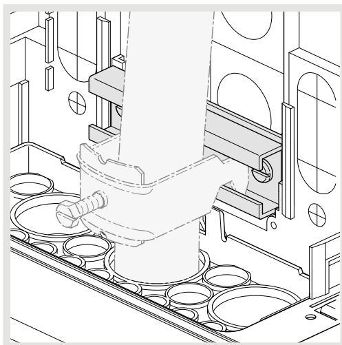
Befestigung von dickem Rohr am Schrank Kunststoff-Fußteil
