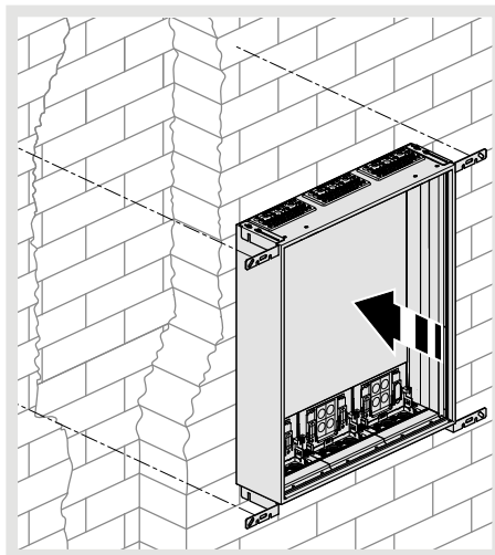
Montage von Befestigungslaschen-Set FZ900 für Unterputz- oder teilversenkten Einbau
