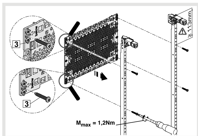
Montage der Kunststoff-Montageplatte UM00M0 auf der Rückseite der univers FW Tragschienen
