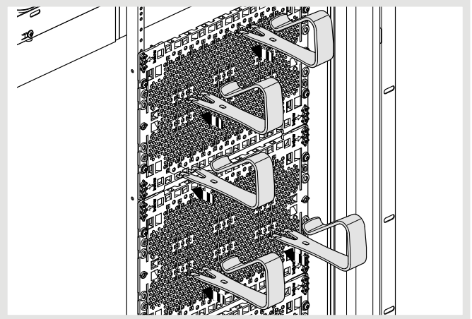
Modemhalter VZ02MM montiert an Kunststoff-Montageplatte UM00M0
