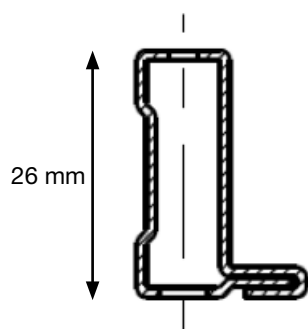
Schnittbild von Univers Z-Tragschiene
