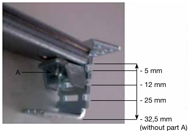
U82A: Hutschiene, absenkbar (200 mm lang) 1-feldig, tiefenverstellbar bis 32,5 mm
