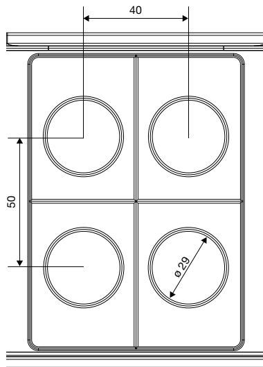
Rückwärtige Leitungseinführungen, im Kunststoff-Kopffußteil
