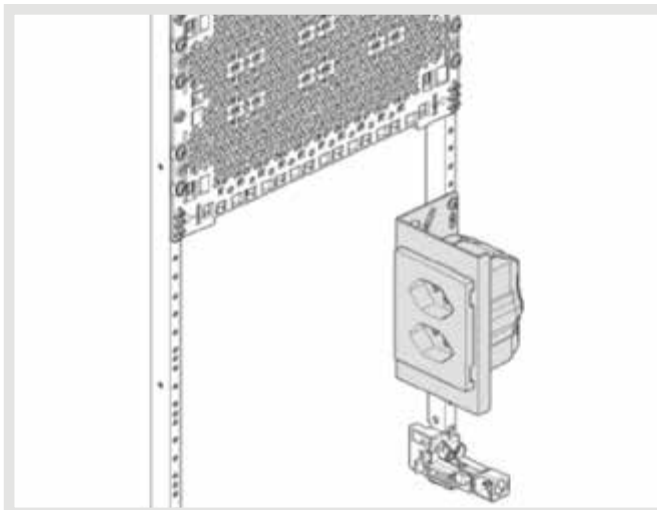
Montage des Steckdosenhalters UM00H0 auf Tragschiene
