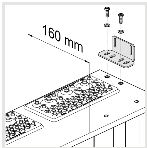
Montage von Befestigungslaschen-Set FZ900H für Unterputz- oder teilversenkten Einbau
