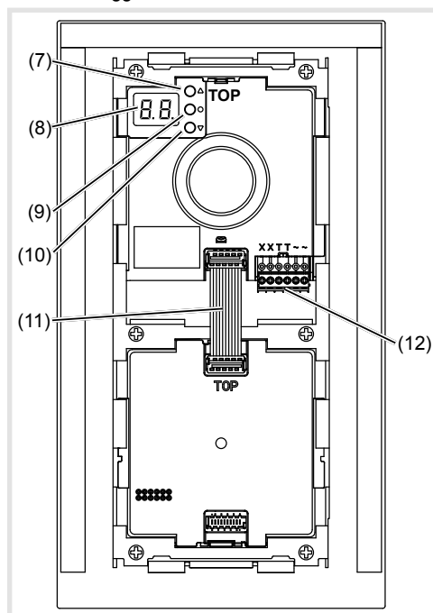
Figura 2: struttura apparecchio, lato posteriore
