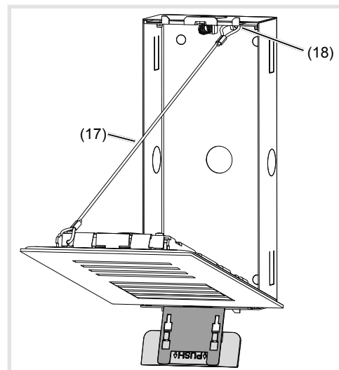
Figura 6: posizione di installazione stazione da porta
