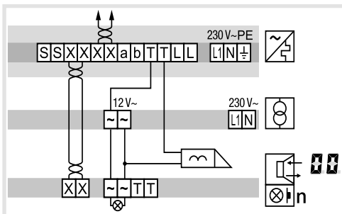
Figura 9: collegamento della stazione da porta con apriporta antimanomissione
