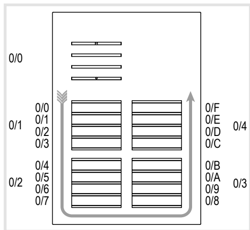
Figura 11: indirizzo modulo e indirizzamento automatico dei tasti di chiamata
