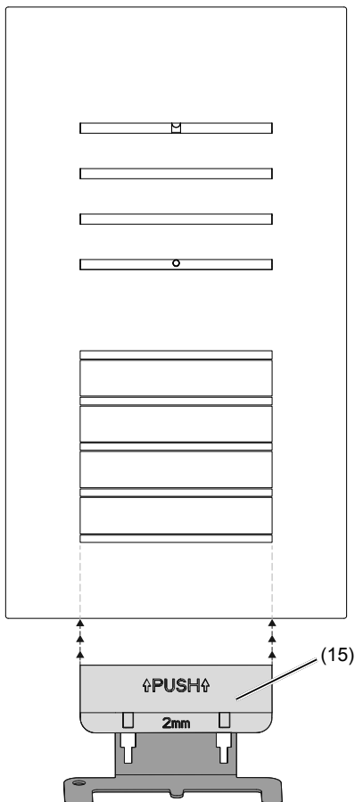
Bild 15: Demontage Türstation
