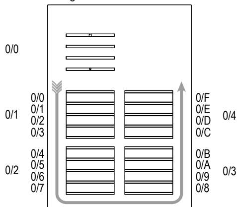
Bild 11: Modul- Adresse und automatische Ruftaster-Adressierung
