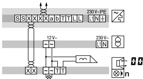
Bild 8: Türöffneranschluss an der Türstation
