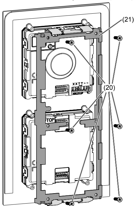
Bild 16: Demontage Modul-Halterung
