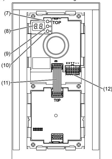
Bild 2: Geräteaufbau Rückseite
