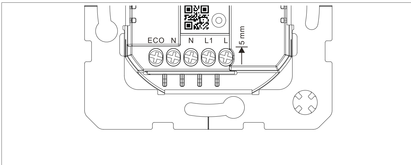
Bild 3: Detailsicht Anschlussklemmen
