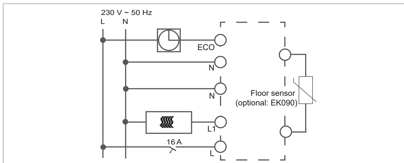
Fig. 6: Collegamento elettrico per il riscaldamento
