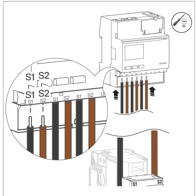
Afbeelding: Een kabelverbinding tot stand brengen
