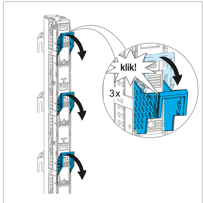
Afbeelding: Het zekeringsschakelaardekse verwijderen
