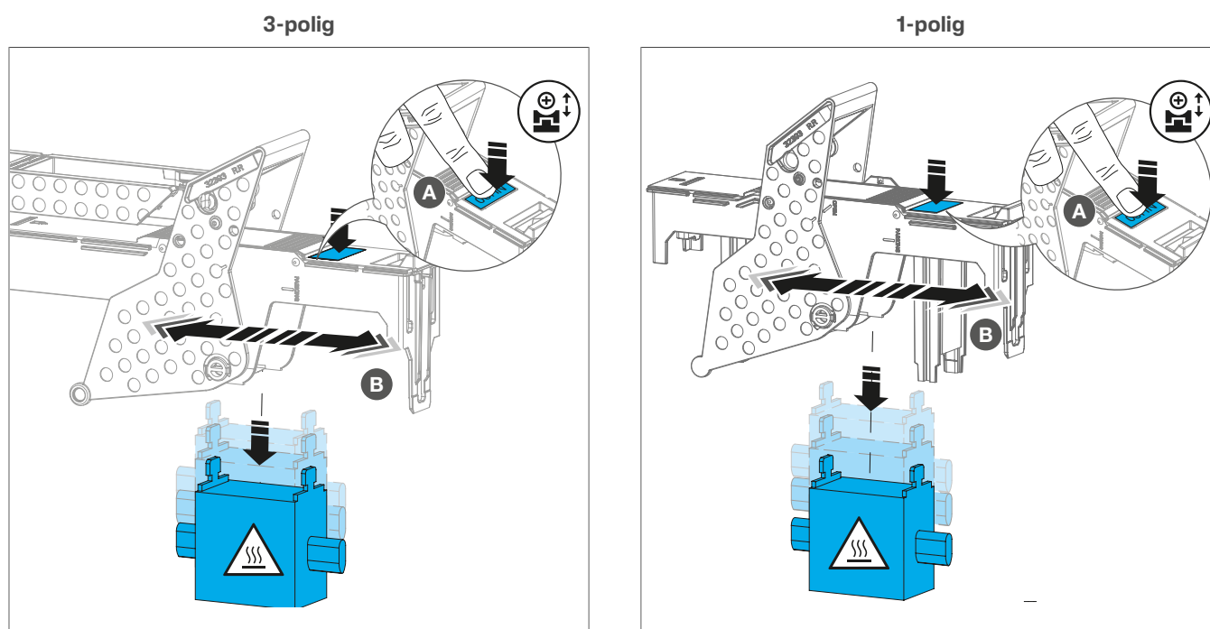
Afbeelding: Zekeringen verwijderen
