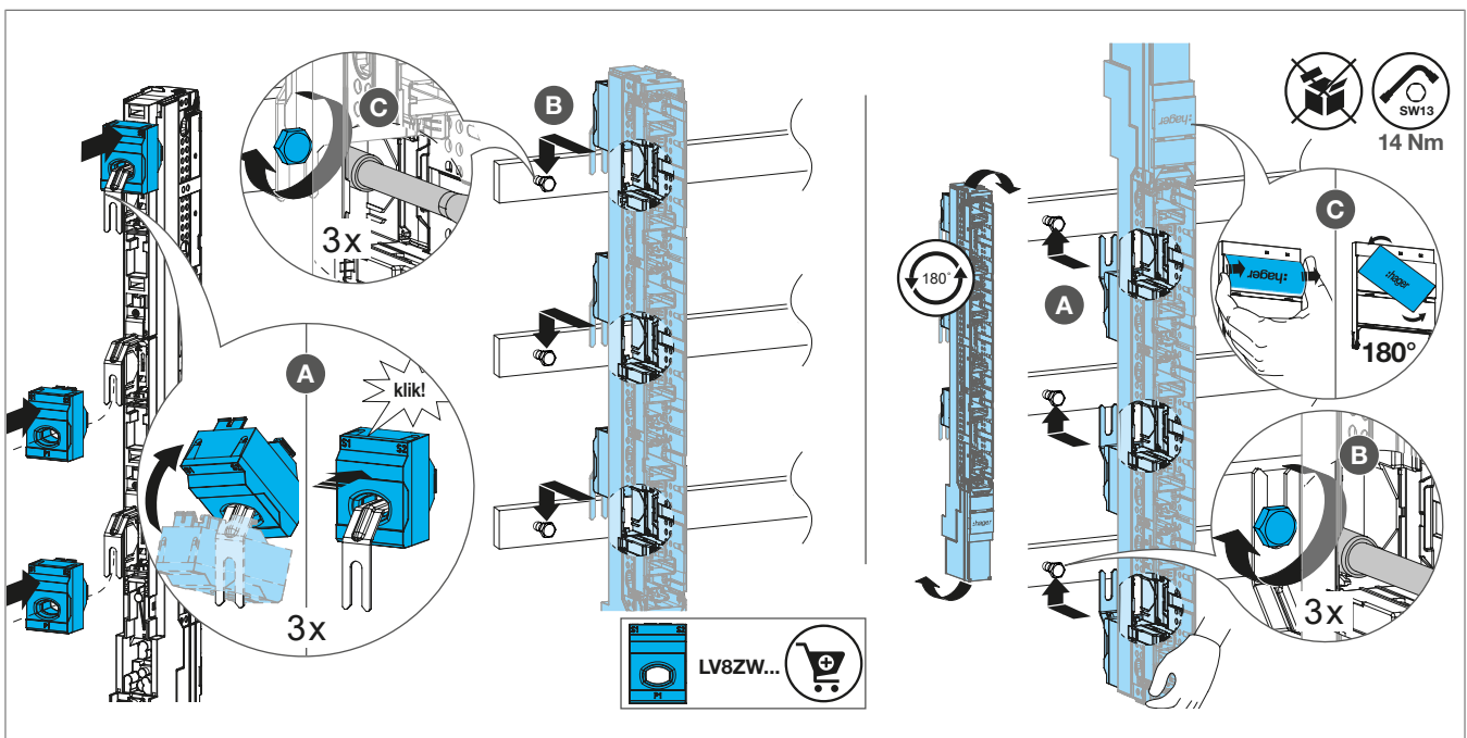
Afbeelding: De stroomtransformatoren installeren met M8-schroeven
