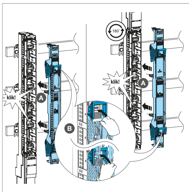
Afbeelding: Het zekeringschakelaardekseel plaatsen en sluiten
