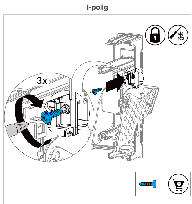
Afbeelding: Het raam vastzetten
