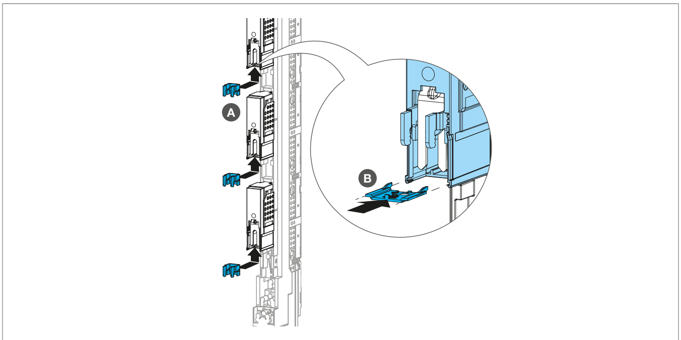
Afbeelding: IP2X-beveiliging monteren (voor installatie met haken)
