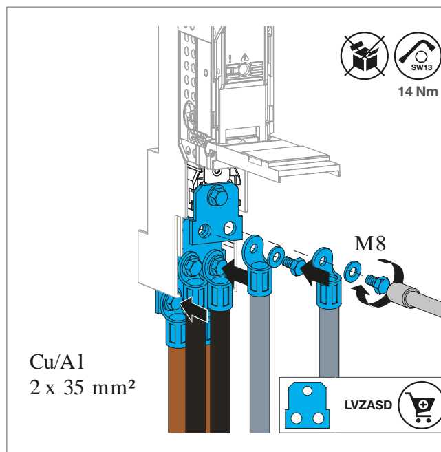
Aansluiting met LVZASD-klemadapter (toeberehen)
