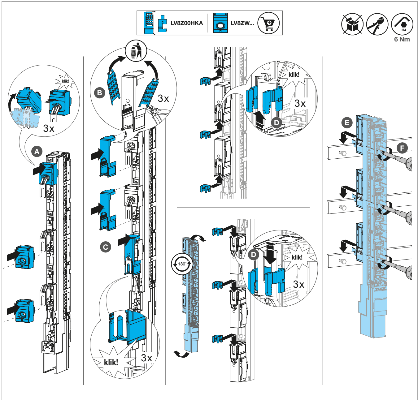
Afbeelding: De stroomtransformatoren installeren met haken
