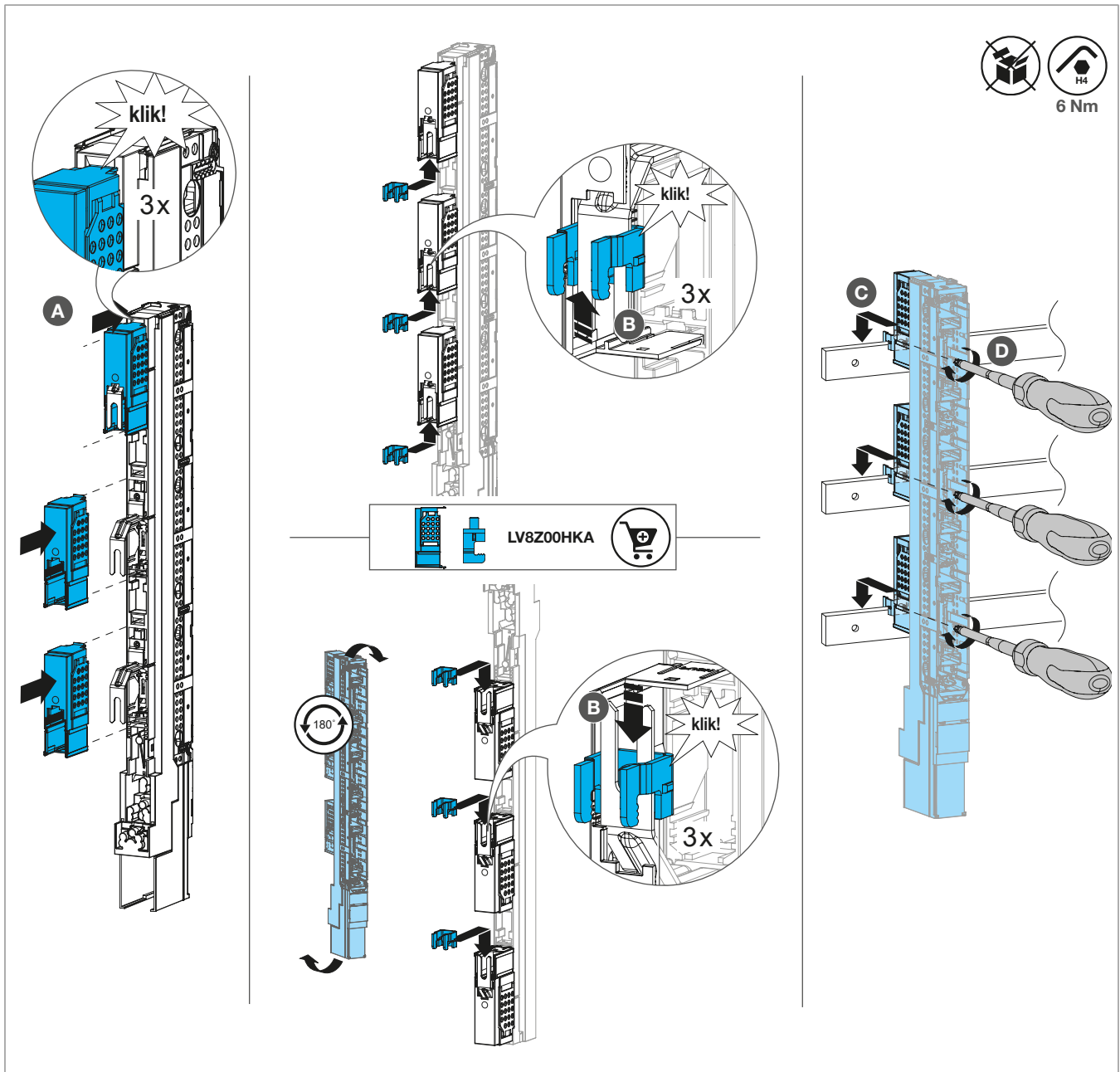
Afbeelding: Installatie met haken
