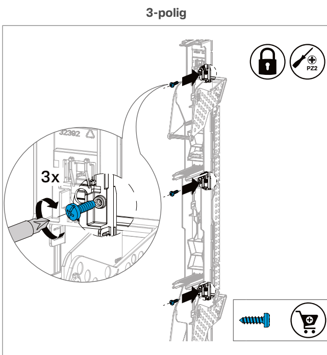
Afbeelding: Het raam vastzetten
