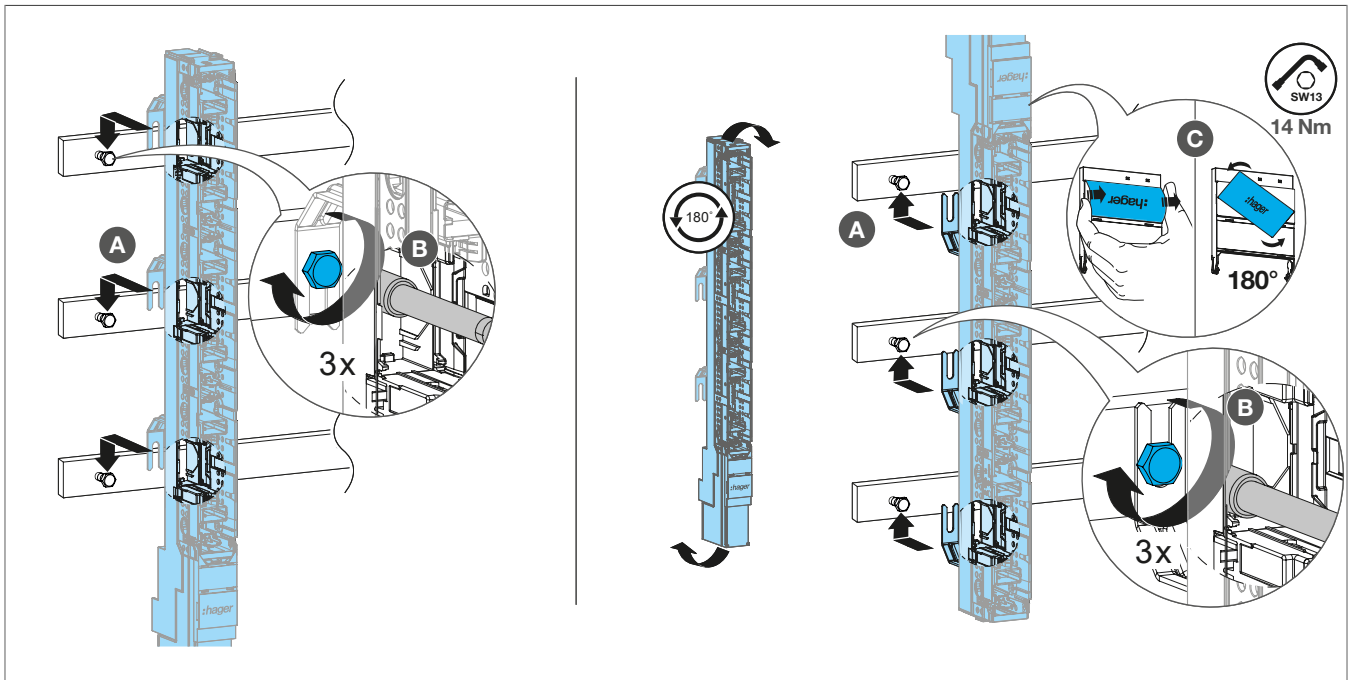
Afbeelding: Vastdraaien van de M8-schroeven
