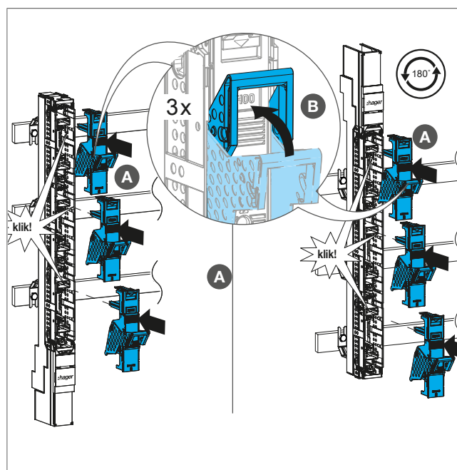
Afbeelding: Het zekeringschakelaardekseel plaatsen en sluiten
