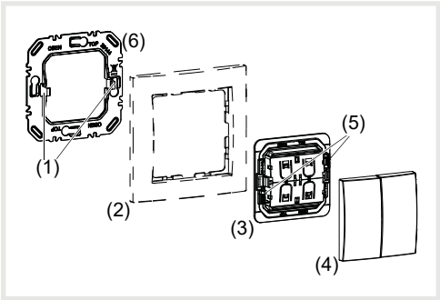
Figura 1: Struttura di principio dell'apparecchio
