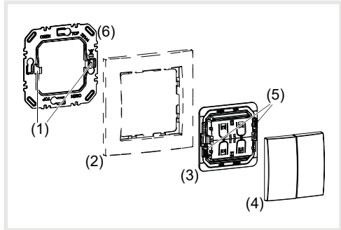
Bild 1: Prinzipieller Geräteaufbau
