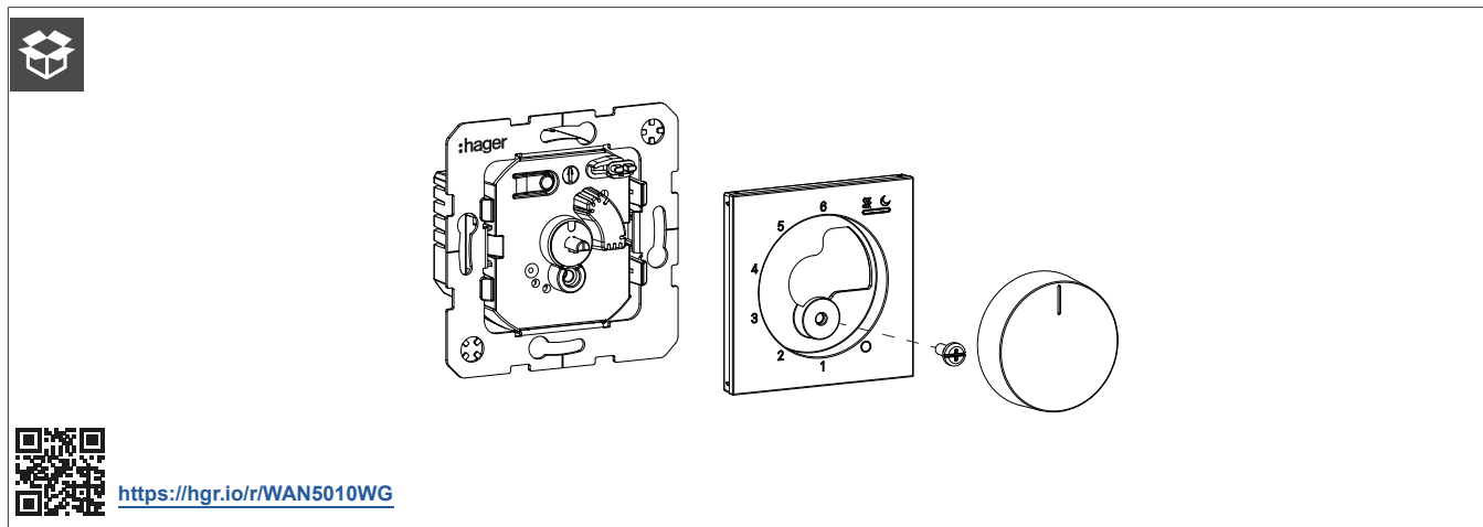
Obraz 1: Dostarczane wyposażenie WAN5010xx
