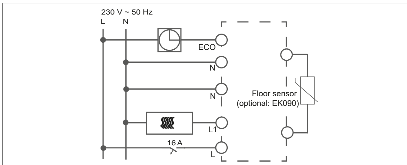
Obraz 7: Połączenie elektryczne ogrzewania
