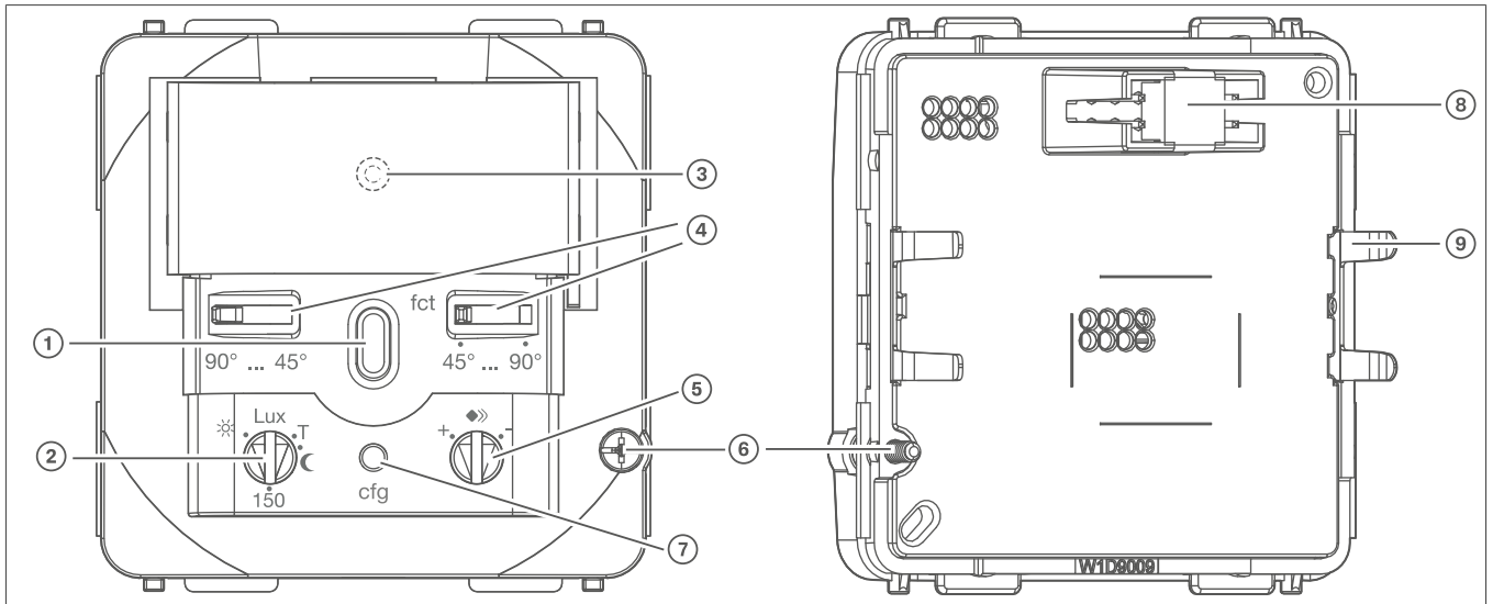
Afbeelding 2: Ontwerp en lay-out van het apparaat
