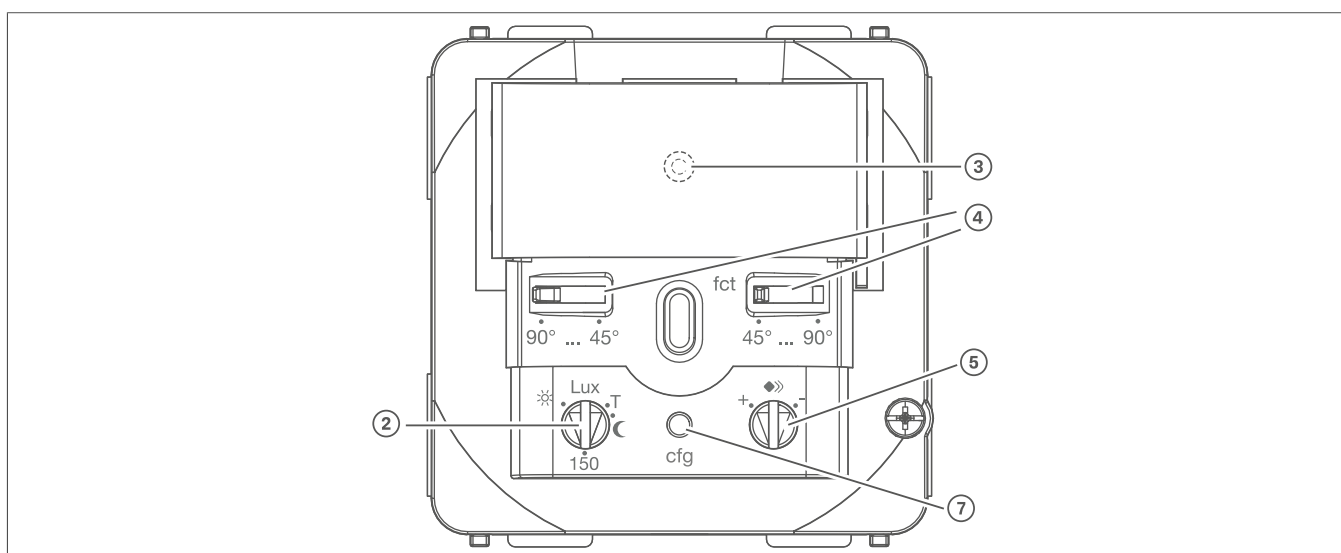
Afbeelding 10: Bedienings- en instelelementen op de opzetmodule.
