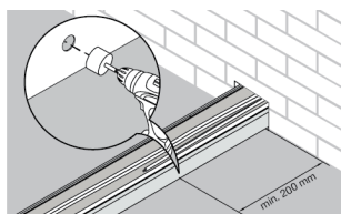
Bohrungen herstellen
