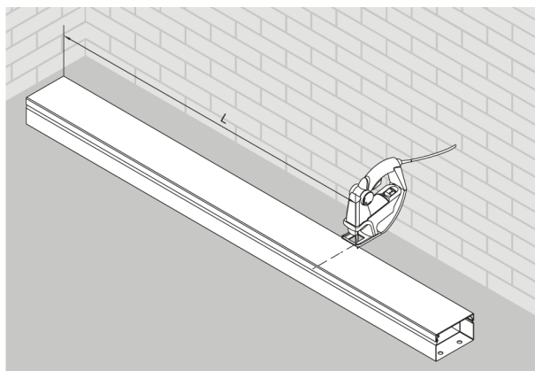
Oberteil beim Ablängen nicht entfernen und bündig ausrichten
