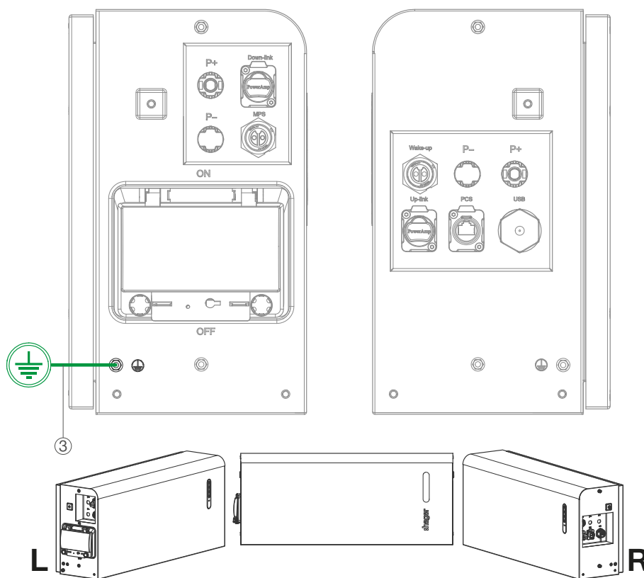
Fig. 28: Connect the PE cable
