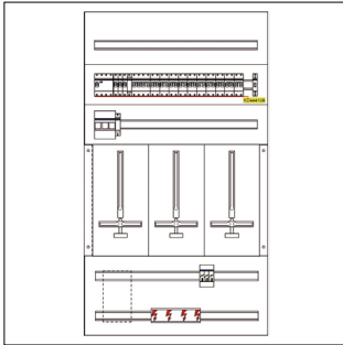
ZW313F-S-002_AUFBAUPLAN_PD
