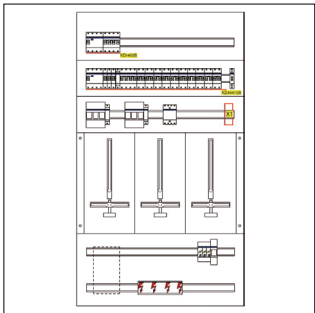
ZW313F-S-012_AUFBAUPLAN_PD
