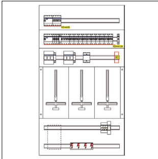
ZW313F-S-012_AUFBAUPLAN_PD
