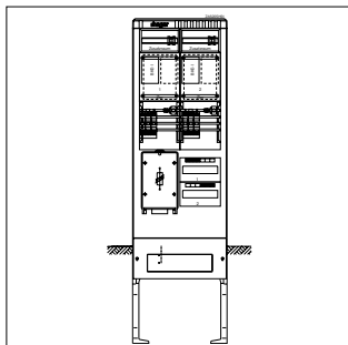
ZAS205HS1
