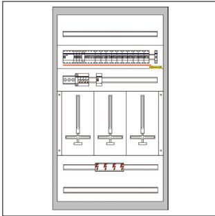
ZW313W-N-003_AUFBAUPLAN_PD
