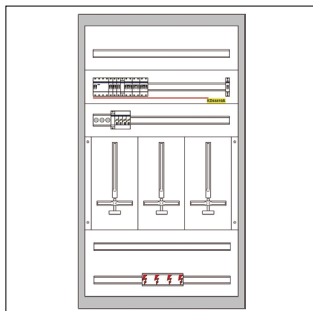
ZW313W-N-005_AUFBAUPLAN_PD
