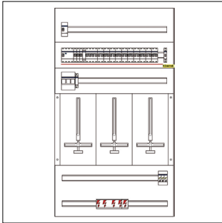
ZW313F-O-004_AUFBAUPLAN_PD
