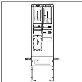
ZAS205BA7
