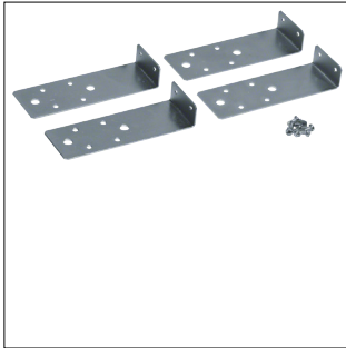
Mauerpratzen,univers, FW, zur Wandmontage des Feldverteiler Unterputz (4 Stück)
