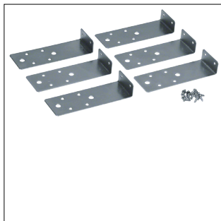
Mauerpratzen,univers, FW, zur Wandmontage des Feldverteiler Unterputz (6 Stück)
