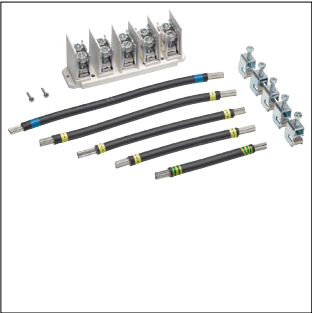
ZM15US
