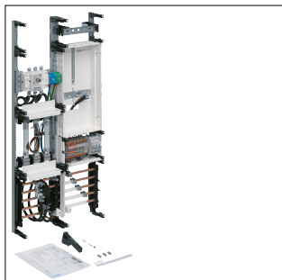
UF32W7N3P_OPEN
