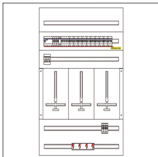
ZW313F-ST-002_AUFBAUPLAN_PD
