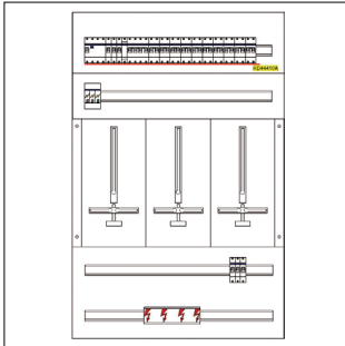
ZW312F-ST-022_AUFBAUPLAN_PD
