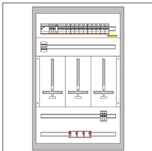
ZW312W-ST-021_AUFBAUPLAN_PD
