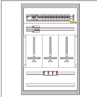
ZW312W-N-021_AUFBAUPLAN_PD
