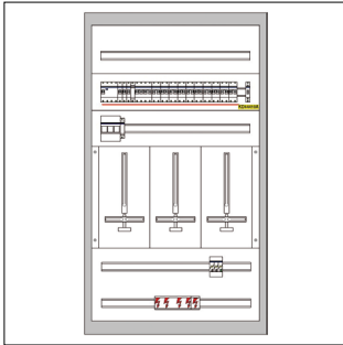
ZW313W-O-001_AUFBAUPLAN_PD
