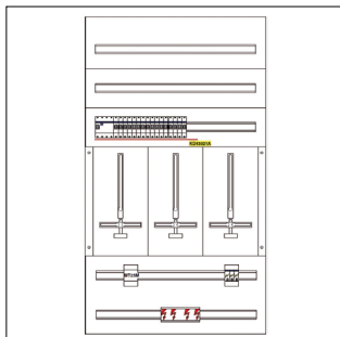
ZW313F-T-002_AUFBAUPLAN_PD
