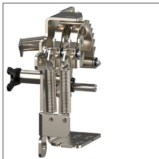
Platine pour interverr.méca. HW1 Débro Couplage (type 3C) - 1 platine/ACB (MI)
