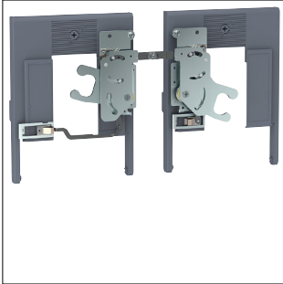
mech. Verriegelungsset 3P x/P630 mit Schaltgestänge (komp. mit Motor+Kipphebel)
