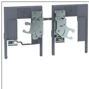
MCCB Zestaw sprzętowy do blokowania jednoczesnego załączenia x630/P630 3P
