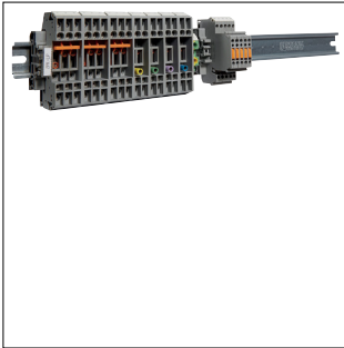
Wandlerprüfklemme 34-pol. mit Hutschiene
