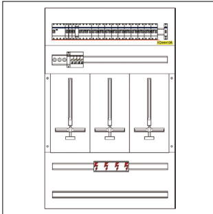
ZW312F-N-022_AUFBAUPLAN_PD
