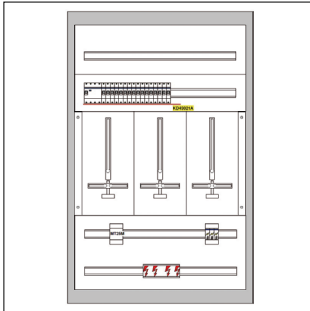
ZW312W-T-021_AUFBAUPLAN_PD
