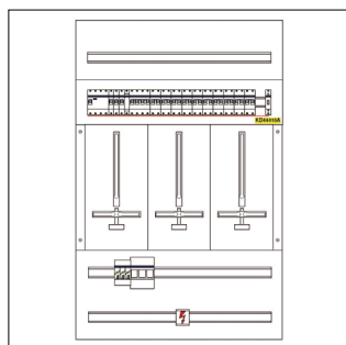
ZW312F-B-022_AUFBAUPLAN_PD
