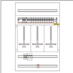
ZW312F-B-022_AUFBAUPLAN_PD
