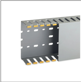
Goulotte de câblage au pas de 20 T1-N 120x60 grise
