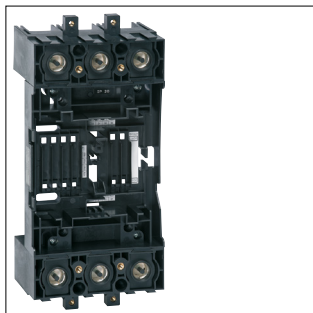
PM base déconnectable h630 LSI 3P (400A)
