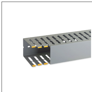
Goulotte de câblage au pas de 20 T1-N 60x100 grise
