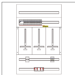
ZW312F-T-022_AUFBAUPLAN_PD
