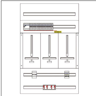
ZW312F-T-022_AUFBAUPLAN_PD
