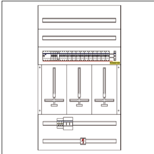
ZW313F-B-002_AUFBAUPLAN_PD
