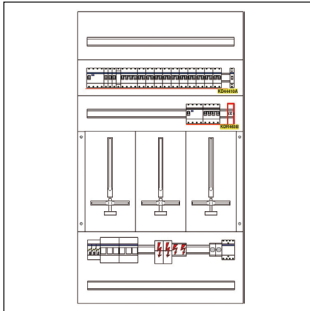
ZW313F-B-012_AUFBAUPLAN_PD
